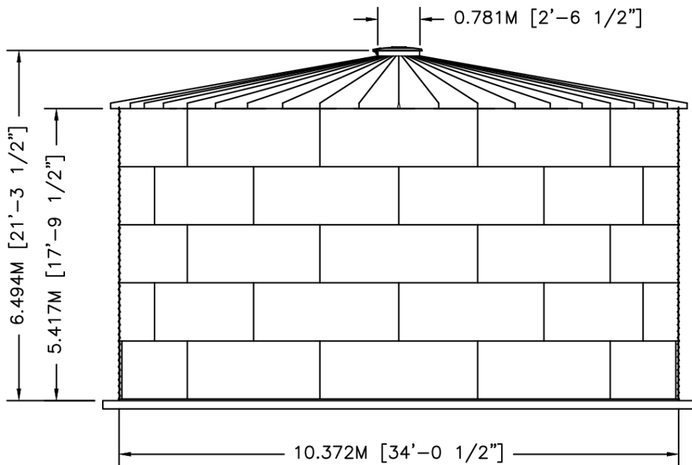
ELEVATION
